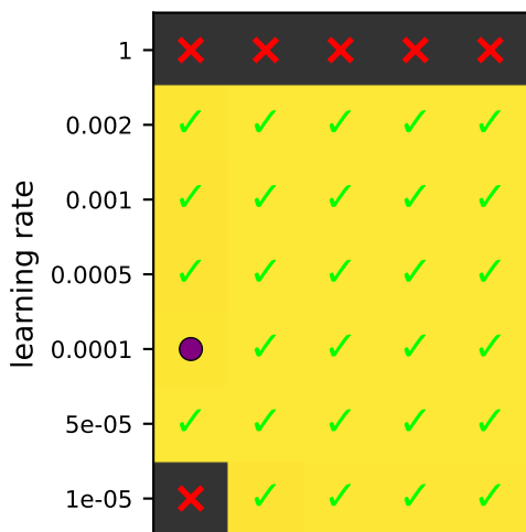
MLP
