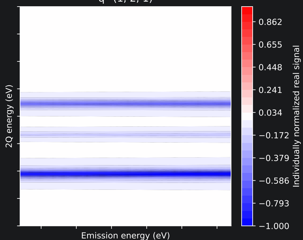
P2: Ku Ku Bu q=(1, 2, 1)
