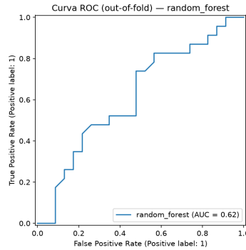
Figura 1: Curva ROC fora-de-dobra do Random Forest (melhor AUC-ROC médio), N=46 .
