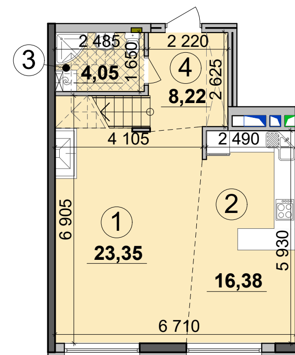
План квартири без перегородок
