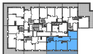
План 26 поверху
