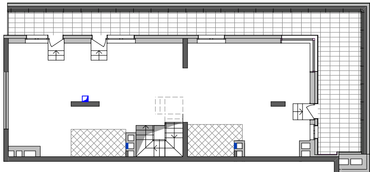
План квартири без перегородок
