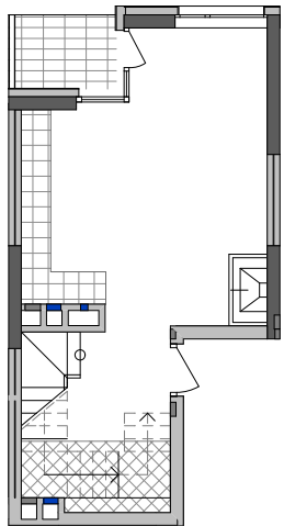
План квартири без перегородок
