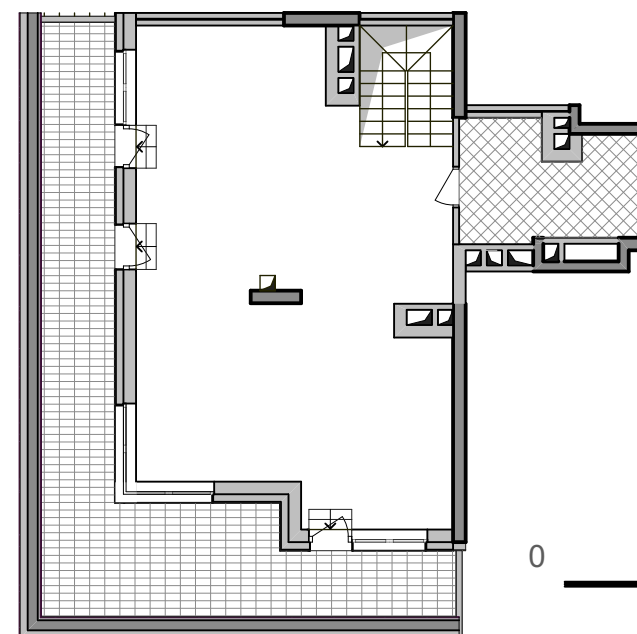
II рівень
