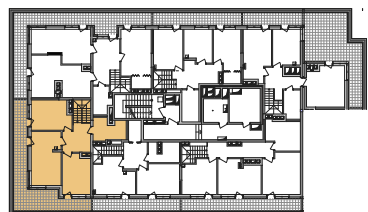
План 25 поверху
