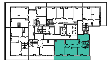
План 26 поверху
