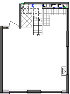
План квартири без перегородок
