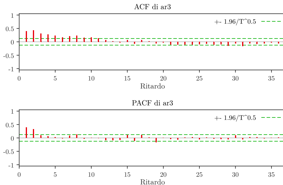
Figura 19 — Autocorrelogramma del modello AR(3): l'ACF decresce lentamente e in modo oscillante, mentre la PACF mostra picchi significativi solo ai primi tre ritardi, coerentemente
