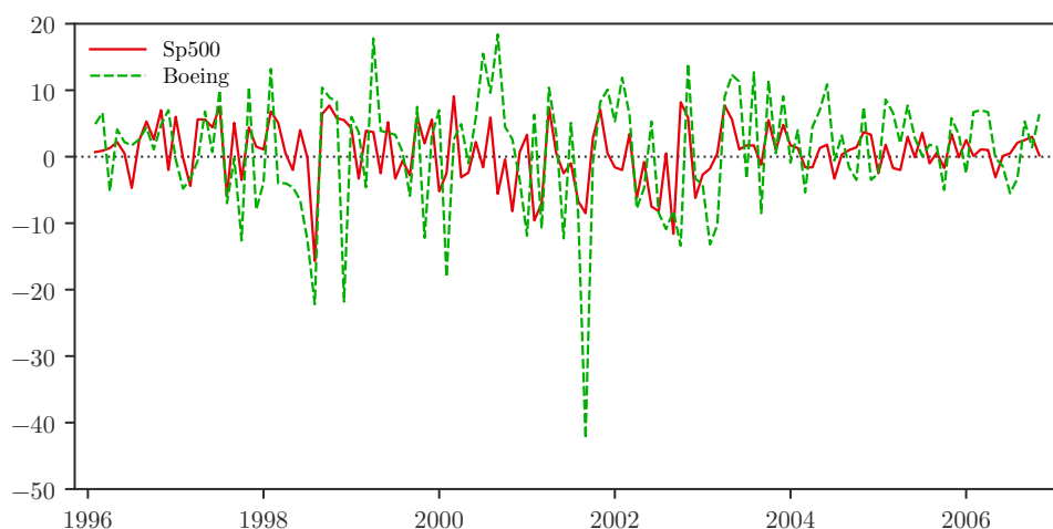
Figura 7 — Serie storiche del rendimento dell'indice Standard & Poor's 500 (portafoglio di mercato) e del titolo rischioso Boeing Co., dal 1996 al 2006: le due serie mostrano un andamento comoviente, con la volatilità di Boeing generalmente amplificata rispetto a quella dell'indice.
