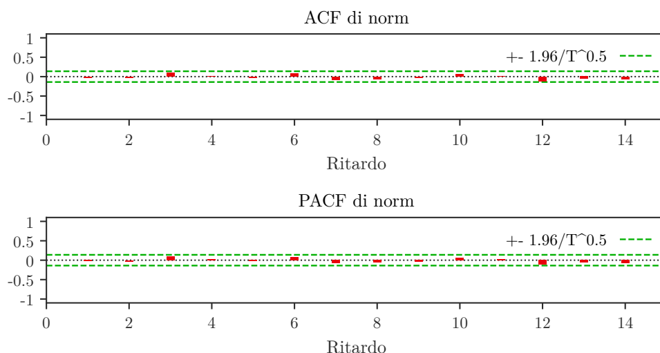
Figura 9 — Grafico dell'autocorrelogramma di un modello White Noise: sia l'ACF che la PACF non mostrano alcun valore significativamente diverso da zero a nessun ritardo, coerentemente con l'assenza di dipendenza seriale.
