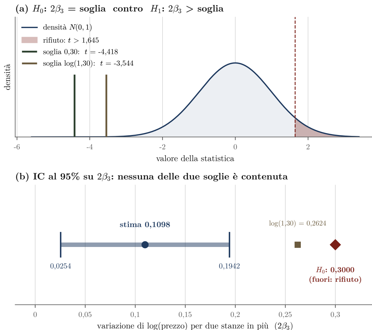
Figura 1.1: Domanda 1. In alto la densità nulla con la regione di rifiuto unilaterale destra e le due statistiche osservate, entrambe lontanissime nella coda opposta; in basso l'intervallo di confidenza al 95% su 2\beta_3 , che esclude sia la soglia approssimata 0,30 sia quella esatta \log(1,30) = 0,2624 .
