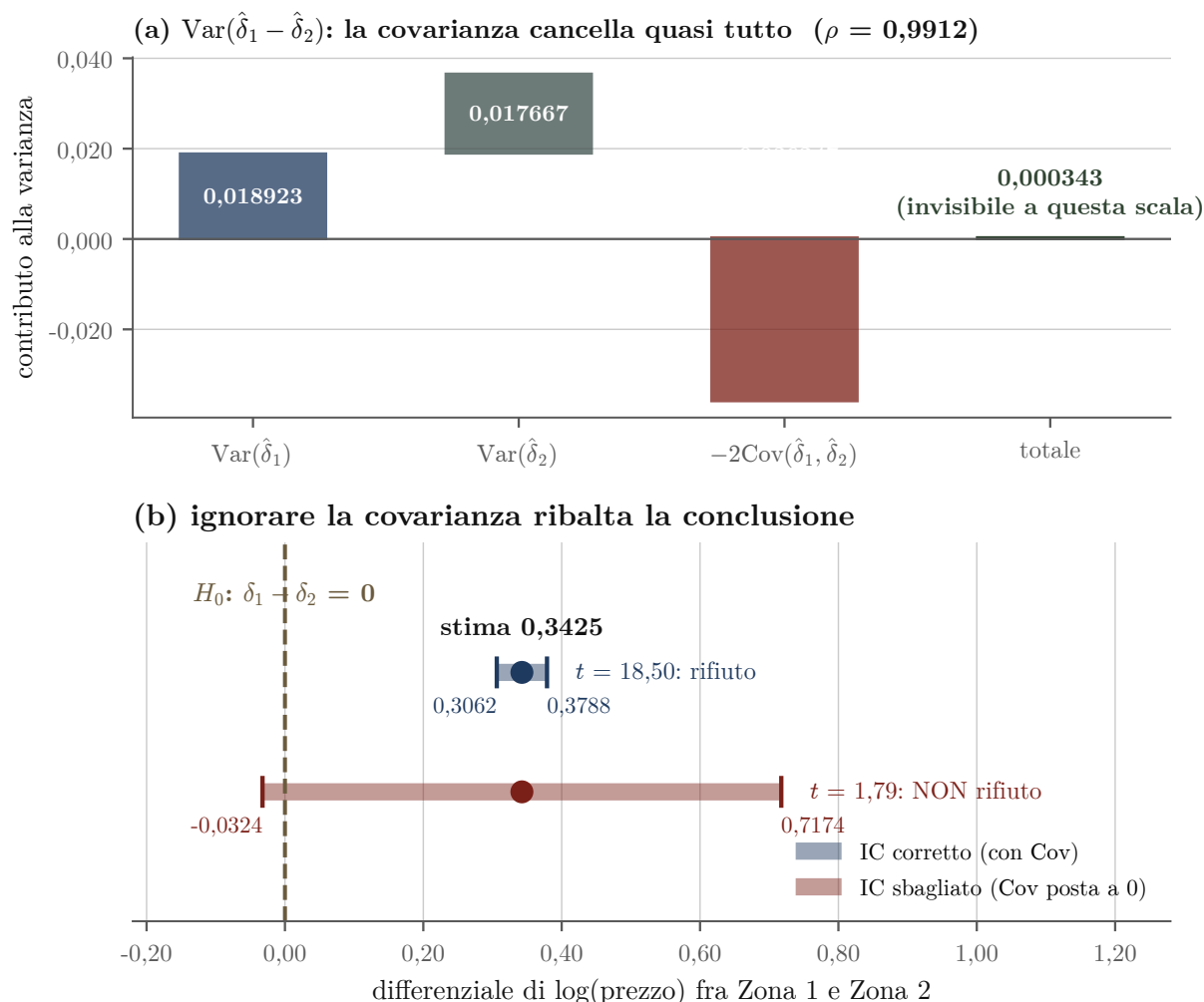
Figura 1.4: Domanda 4. In alto la varianza del differenziale scomposta termine per termine: le due varianze si sommano a 0,036590, ma -2 \text{Cov} ne sottrae 0,036247, lasciando un residuo di 0,000343 invisibile alla scala del grafico. In basso il confronto fra l'intervallo corretto e quello che si otterrebbe ponendo erroneamente la covarianza a zero: il primo esclude nettamente lo zero, il secondo lo contiene.
