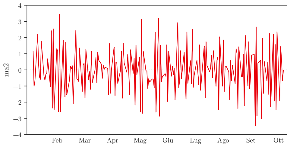
Figura 14 — Grafico di una serie storica di un modello MA(2) con \theta_1 = -0.9, \theta_2 = 0.7, \sigma = 0.9 : la serie mostra oscillazioni più regolari rispetto al MA(1), riflesso della dipendenza da due shock passati.
