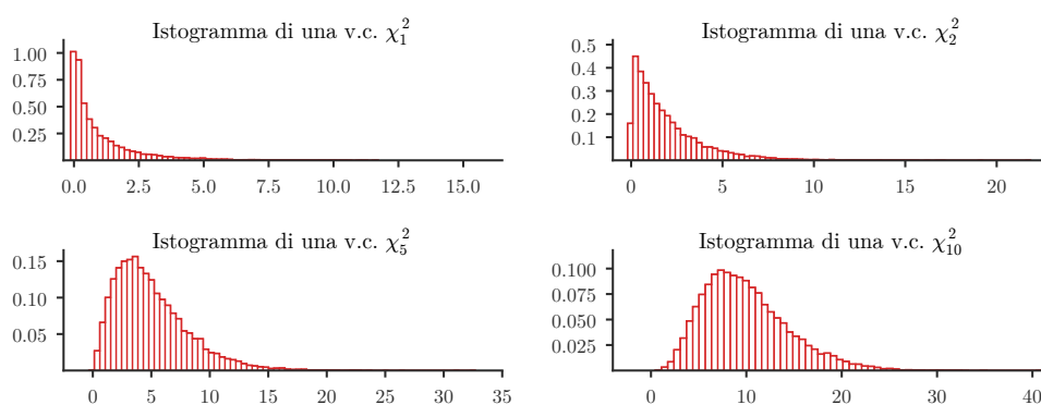
Figura 2 — \chi_{df}^2 con diversi gradi di libertà, cioè df = 1, 2, 5, 10 . Il pannello mostra quattro istogrammi di variabili casuali chi-quadro simulate con gradi di libertà crescenti (1, 2, 5, 10): per df = 1 la densità è fortemente concentrata vicino allo zero e decrescente; all'aumentare dei gradi di libertà la distribuzione si sposta verso destra, si allarga e assume una forma progressivamente più simmetrica e campanulare, illustrando visivamente come l'approssimazione chi-quadro della F migliori (in forma) al crescere dei gradi di libertà al denominatore. (slide 15)
