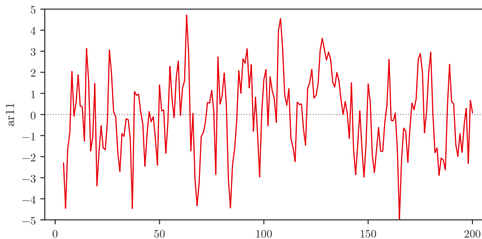
Figura 16 — Grafico di una serie autocorrelata al primo ordine: la serie oscilla con maggiore persistenza rispetto al white noise, alternando fasi più prolungate sopra e sotto lo zero.
