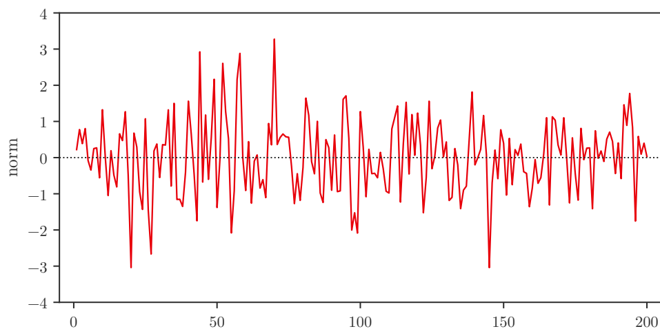
Figura 8 — Esempio di dati generati da un modello White Noise: la serie oscilla in modo irregolare attorno a zero, senza pattern visibile, con ampiezza compresa circa tra -4 e 4 .
