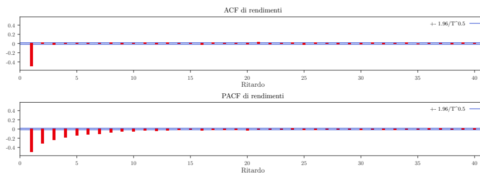
Figura 13 — Struttura di autocorrelazione (ACF e PACF) dei rendimenti calcolati sui dati di Figura 12: si osserva un unico valore negativo significativo al ritardo 1 nell'ACF, in linea con quanto atteso per un modello MA(1); la PACF mostra invece una struttura decrescente su più ritardi, tipica della rappresentazione AR di un processo MA.
