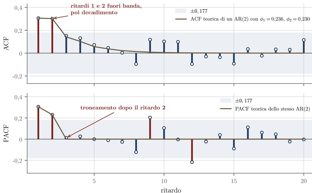
Figura 1.8: ACF e PACF di Delta \log(\text{usa}) lette sulla Figura 3 dell'esame (p. 4), riprodotta in testa alla domanda, con le bande a più o meno 0,177 , sovrapposte all'ACF e alla PACF teoriche dell'AR(2) identificato per inversione di Yule-Walker, con \phi_1 pari a 0,236 e \phi_2 pari a 0,230 .
