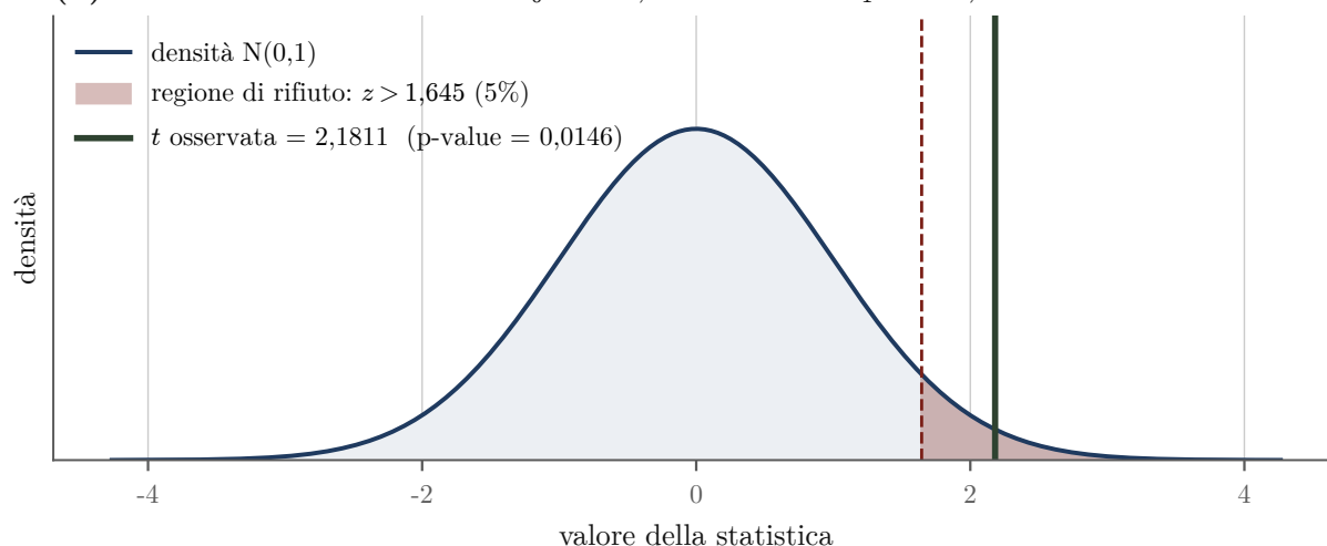
Figura 7.1: Sopra: l'intervallo di confidenza al 95% per \theta = 30\beta_4 su una retta numerica; entrambe le soglie candidate (0,0200 e \log(1,02) = 0,0198 ) cadono alla sinistra dell'estremo inferiore 0,0224. Sotto: la densità N(0,1) sotto H_0 con la regione di rifiuto unilaterale destra al 5% e la statistica osservata t = 2,1811 .
