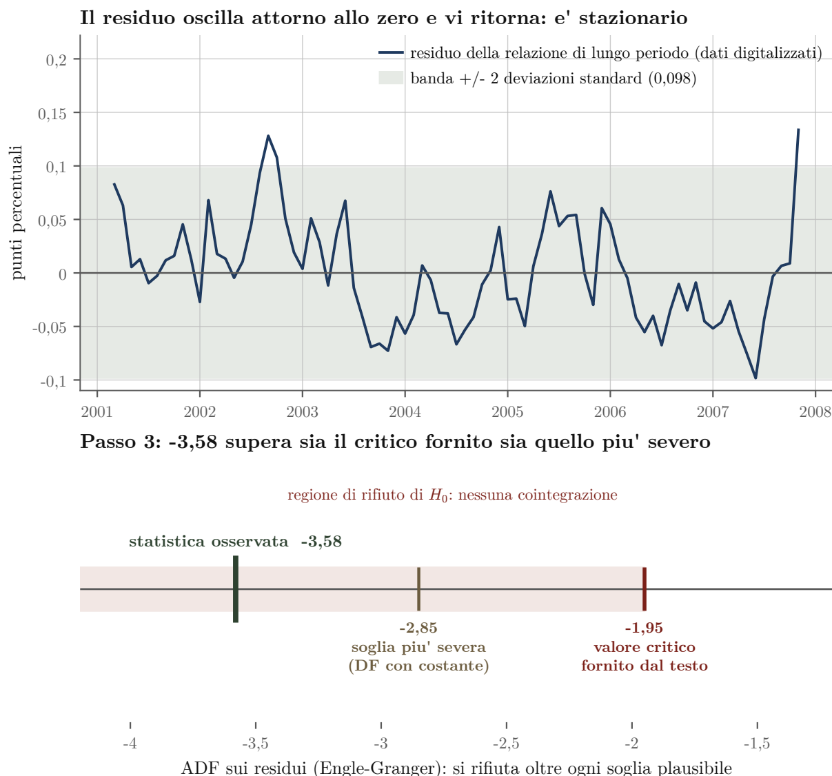
Figura 6.3: Sopra: il residuo della relazione di lungo periodo calcolato sui dati digitalizzati dalla Figura 1, che oscilla attorno allo zero dentro una banda di due deviazioni standard senza allontanarsene. Sotto: la statistica osservata -3,58 confrontata con il valore critico fornito dal testo e con la soglia piu' severa delle note.
