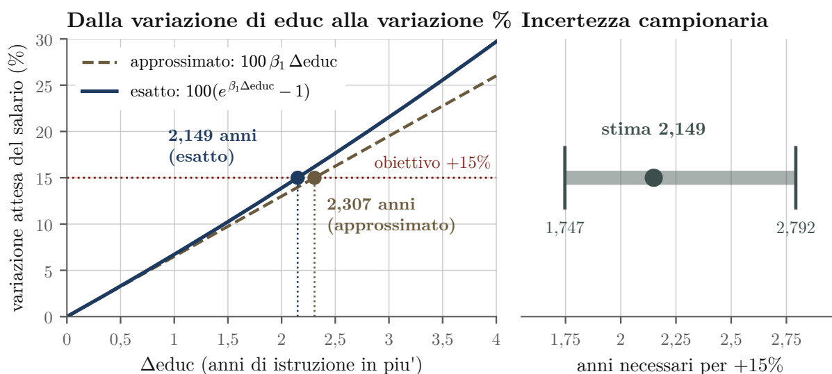
Figura 9.1: Sinistra: la percentuale attesa di variazione del salario in funzione di \Delta\text{educ} , nella versione approssimata (tratteggio) e in quella esatta (linea continua); la riga orizzontale è l'obiettivo del 15 per cento e i due punti marcati sono le due soluzioni, 2,307 e 2,149 anni. Destra: l'intervallo di confidenza al 95 per cento del numero di anni, ottenuto propagando l'intervallo di \beta_1 . Dati veri ricalcolati, n = 722 .
