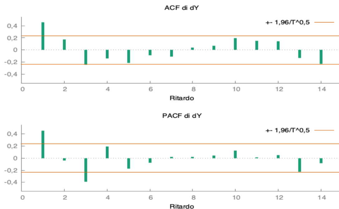
Figura 12.5: Figura 2 del tema d'esame: «ACF e PACF della serie \Delta gfr ». Riprodotta dall'originale; correlogramma ACF (in alto) e PACF (in basso) della serie dY , su 14 ritardi, con le bande \pm 1,96/\sqrt{T} .
