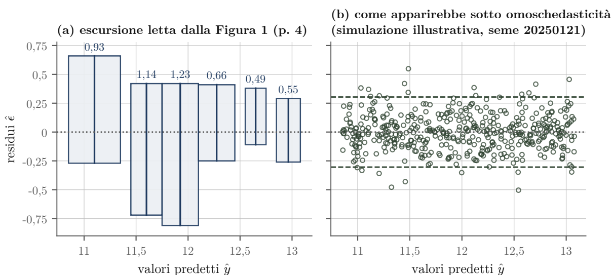
Figura 13.7: Domanda 6. A sinistra l’escursione dei residui per fascia di valori predetti, letta a occhio sulla Figura 1 del tema, riprodotta sopra (p. 4): l’ampiezza passa da circa 1,2 nella parte centrale a circa 0,5 a destra. A destra, per confronto, come apparirebbe una nube genuinamente omoschedastica con la stessa numerosità: una banda di larghezza costante (simulazione illustrativa, seme 20250121).
