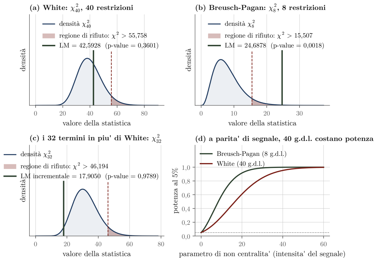
Figura 11.4: Pannelli (a), (b), (c): le tre distribuzioni nulle con la statistica osservata e la regione di rifiuto al 5%: White non rifiuta, Breusch-Pagan rifiuta, e il test incrementale sui 32 termini non lineari cade a sinistra della moda. Pannello (d): a parità di intensità del segnale, la potenza del test a 8 gradi di libertà domina quella del test a 40.
