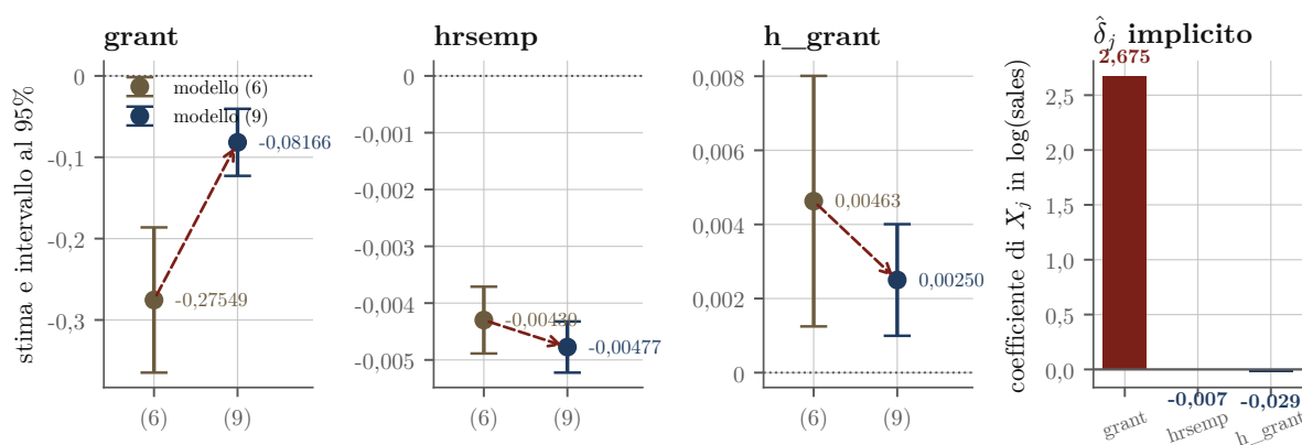
Figura 4.5: Tre pannelli a sinistra: stime e intervalli di confidenza al 95 per cento dei coefficienti di grant , hrsemp e h_grant nel modello (6) e nel modello (9), con la freccia che indica lo spostamento. Pannello a destra: coefficienti impliciti della regressione ausiliaria di \log(\text{sales}) sui regressori del modello corto, ricavati dividendo lo spostamento per il coefficiente di l_sales .
