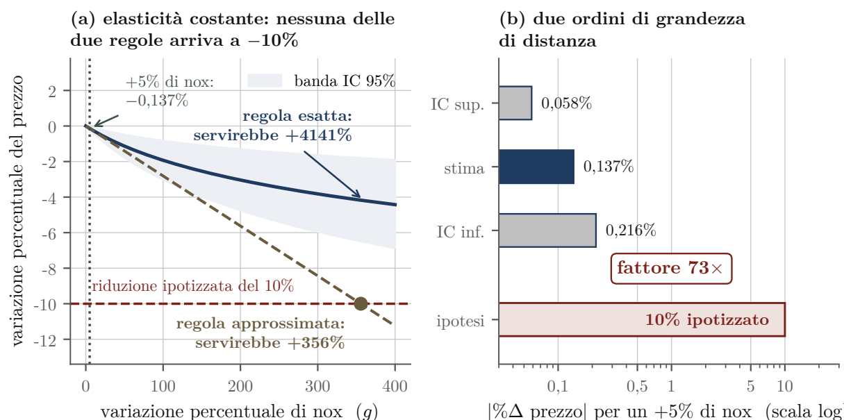
Figura 13.3: Domanda 3. A sinistra la variazione percentuale del prezzo in funzione di quella di nox: la curva esatta (blu) con la sua banda al 95% e la regola lineare approssimata (ambra). Nessuna delle due tocca il -10% per un aumento del 5%; la riga rossa mostra quanto sarebbe lontano l'obiettivo. A destra il confronto di ordine di grandezza su scala logaritmica: fra l'effetto stimato di un +5% e il -10% ipotizzato corre un fattore 73.
