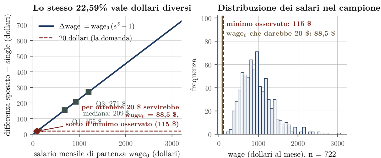
Figura 9.2: Sinistra: la differenza in dollari fra sposato e single implicata dal modello, wage_0(e^\delta - 1) , in funzione del salario di partenza; i quadrati segnano i quartili del campione e la retta orizzontale il valore di 20 dollari chiesto dalla domanda. Destra: la distribuzione dei salari mensili osservati; una riga segna il minimo (115 dollari), l'altra il livello di 88,5 dollari che sarebbe necessario perché la differenza fosse di 20 dollari. Dati veri ricalcolati, n = 722 .
