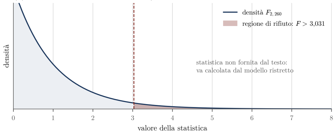
(a) H_0 : \beta_1 = \beta_2 = 0 — densità' F_{2, 260} e regione di rifiuto al 5%
