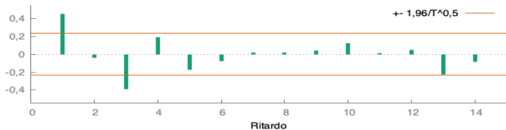
PACF di dY
