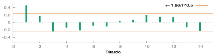
ACF di dY
