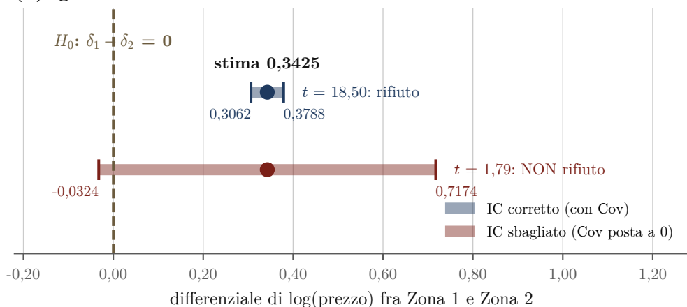
(b) ignorare la covarianza ribalta la conclusione
