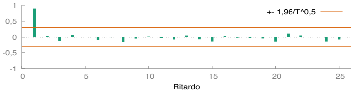
PACF di lprice
