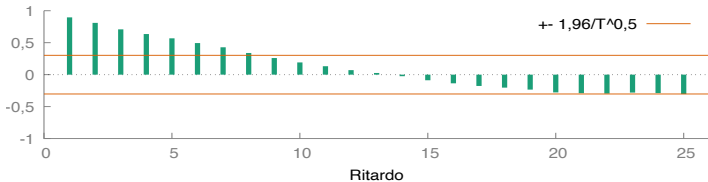
ACF di lprice
