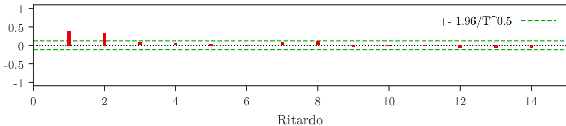
PACF di ar3
