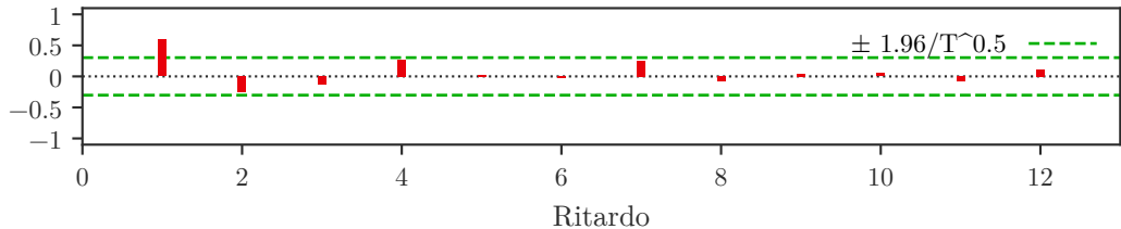
PACF di linvpc
