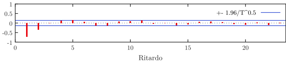
PACF di ma2
