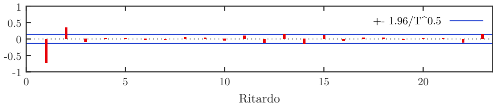
ACF di ma2
