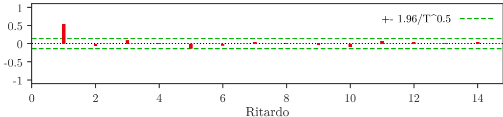
PACF di ar11
