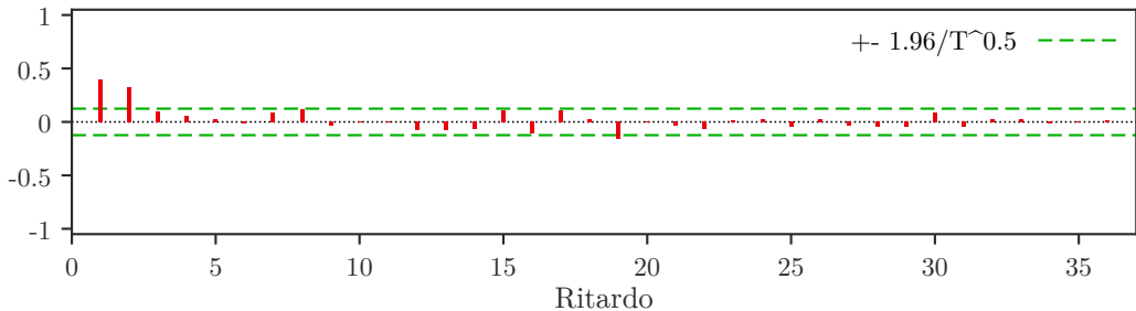
PACF di ar3
