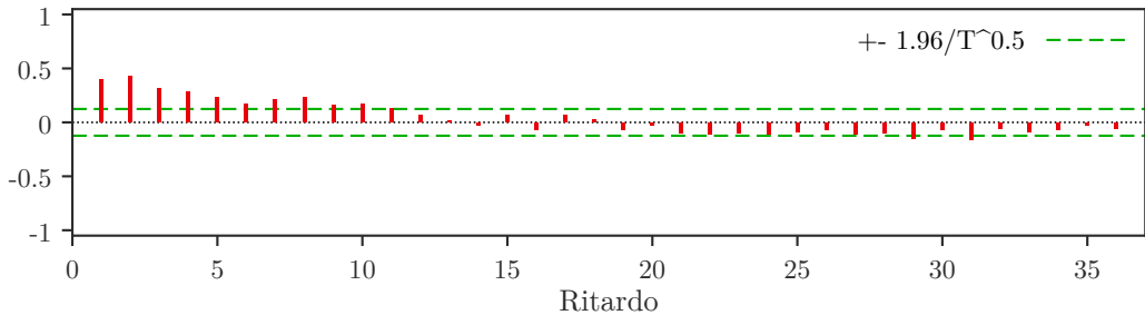
ACF di ar3
