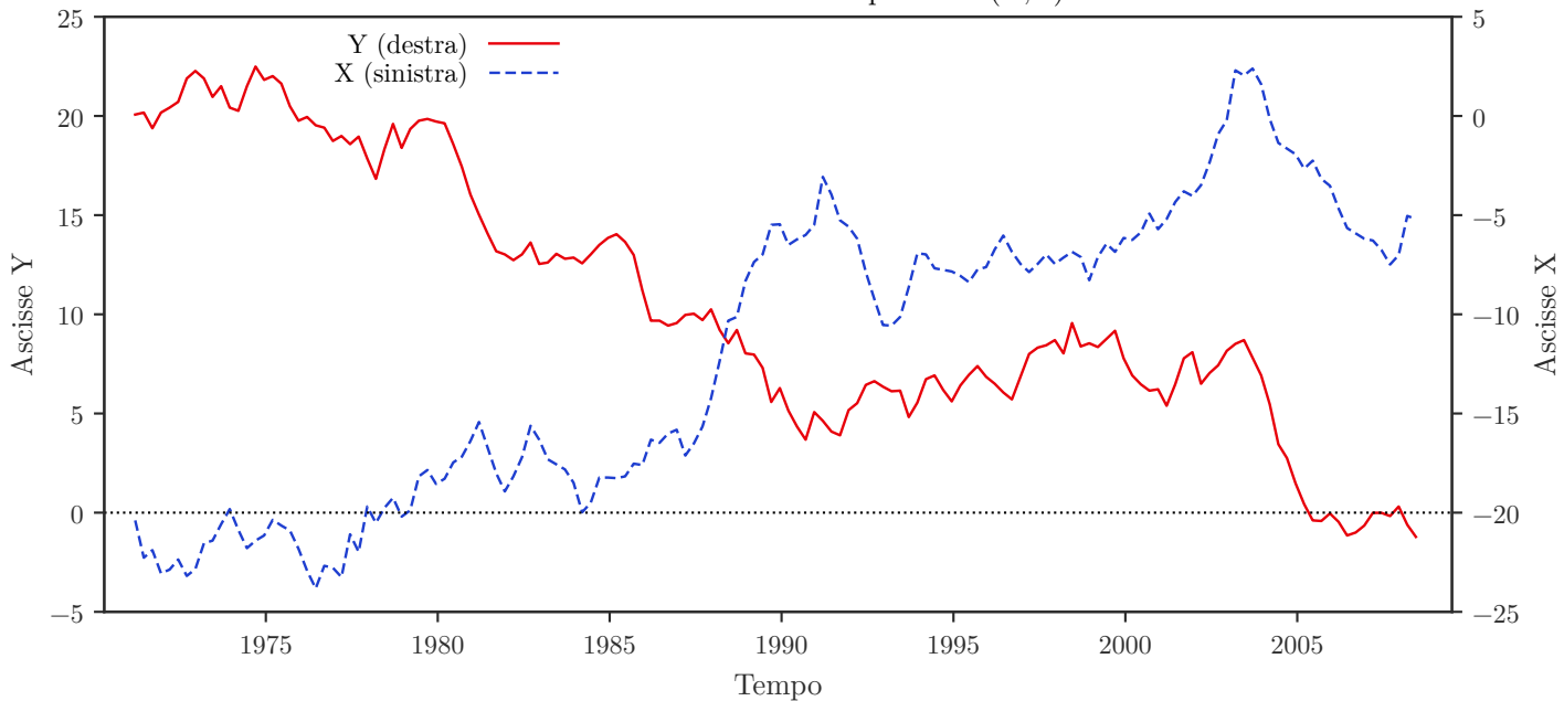
Grafico dei random walk indipendenti (Y,X)
