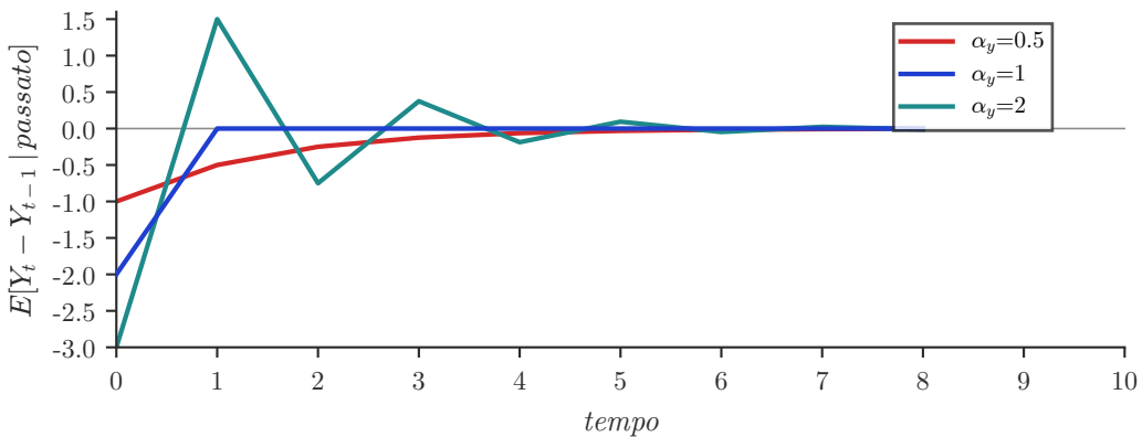
Andamento di E[\Delta Y_t | \text{passato}] per diversi valori di \alpha_y
