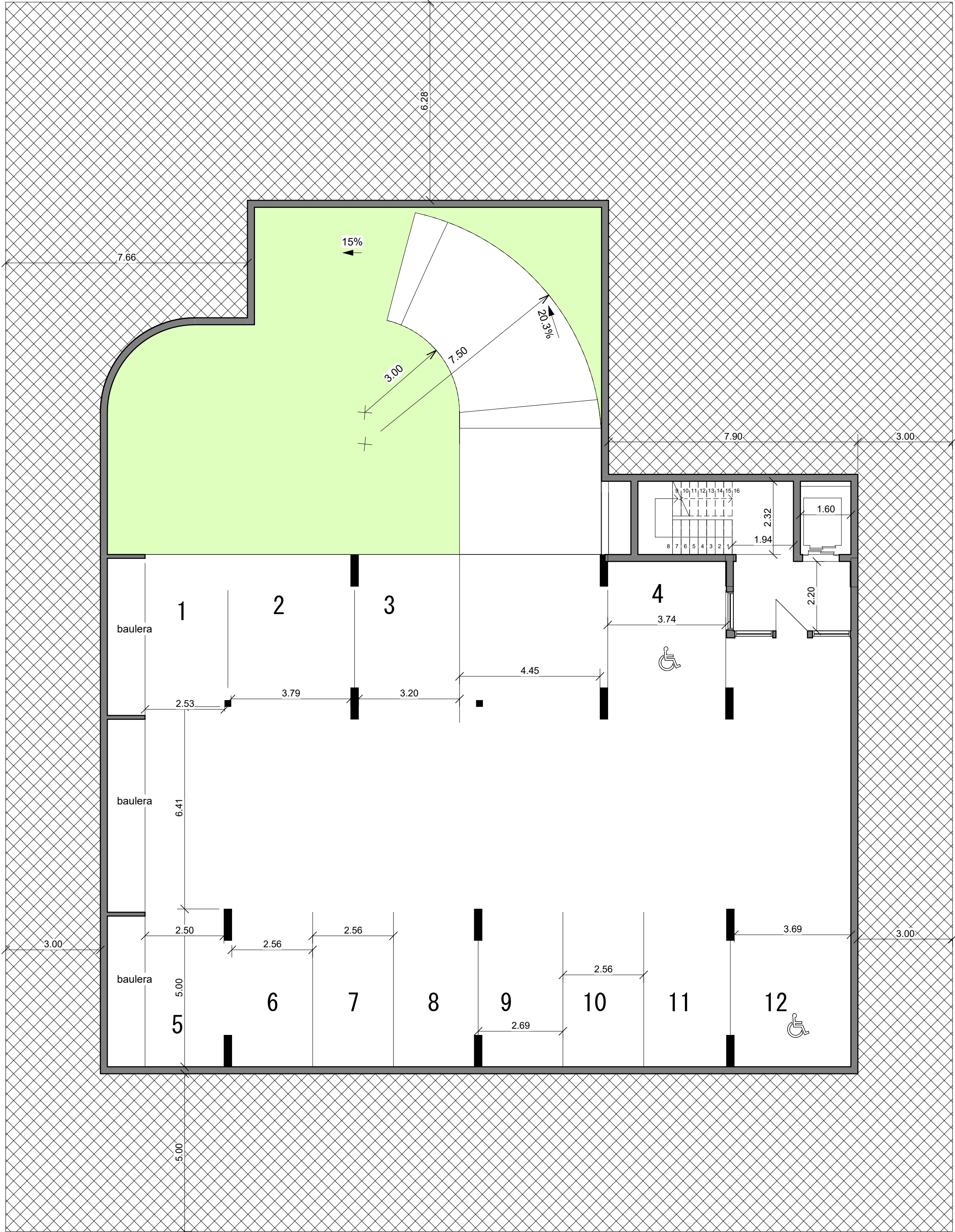
1 SUBSUELO L03 1 : 100
