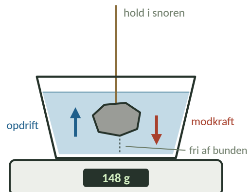
Figur 1: Sådan måles rumfanget. Vægten nulstilles med vandskålen på (1). Når stenen hænger frit i vandet, viser vægten massen af det vand, stenen fortrænger (2).
