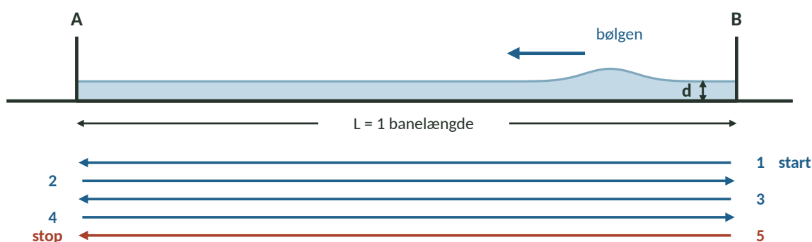
Figur 2: Opstillingen. Ende A løftes, og vandet samler sig i ende B (1). Når karret sættes ned, løber bølgen frem og tilbage, og I tager tid på fem banelængder (2).
