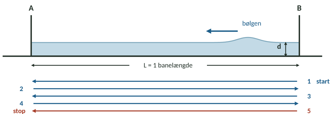
Figur 2: Opstillingen. Ende A løftes, og vandet bliver dybest i ende B (1). Når karret sættes ned, løber bølgen frem og tilbage, og I tager tid på fem banelængder (2).
