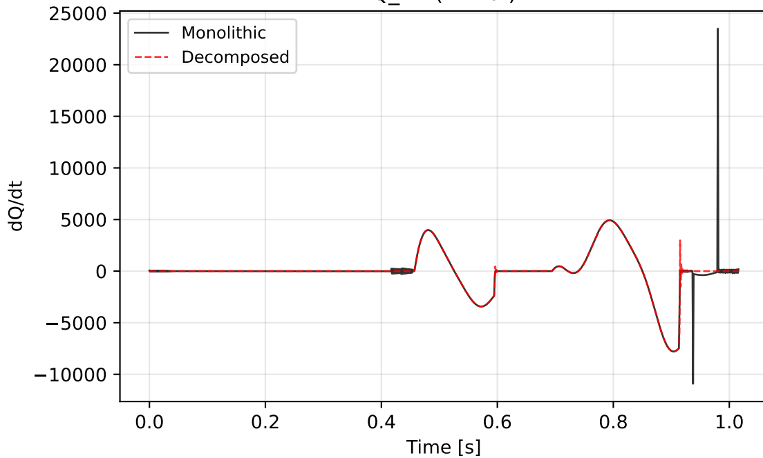
Q_LA (mitral)
