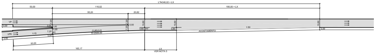
NARIZ TIPO 6 RAMO DE ENTRADA DE 2 FAIXAS
