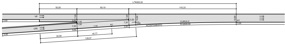
NARIZ TIPO 5 RAMO DE ENTRADA DE 2 FAIXAS
