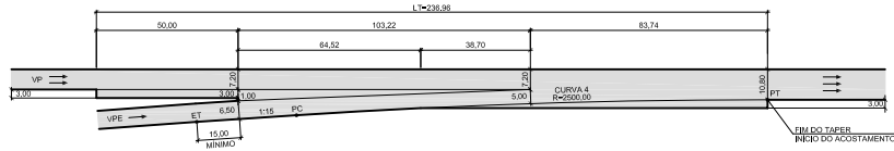
NARIZ TIPO 4 RAMO DE ENTRADA DE 1 FAIXA
