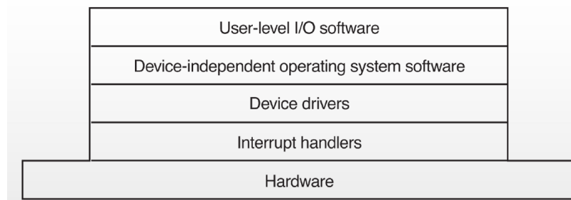
Figure 13.12: Stratificazione I/O
