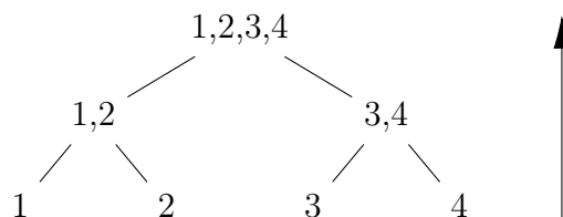
Figure 7.1: Fase di up-sweep sull'albero bilanciato.
