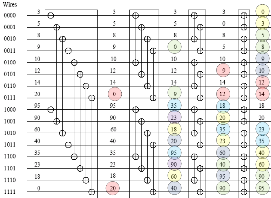
Figure 7.5: Esempio di rete bitonica per n = 16 .
