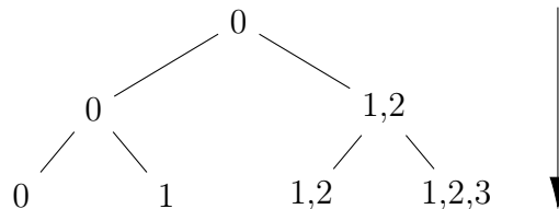
Figure 7.2: Fase di down-sweep sull'albero bilanciato.
