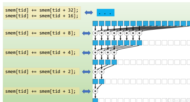
Figure 3.1: Uso dei thread del warp per il loop unrolling
