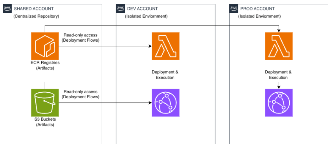
Figura 8: Topologia della strategia Multi-Account su AWS. L'account Shared centralizza gli artefatti, referenziati in sola lettura per il deployment negli ambienti isolati [Elaborazione dell'autore].
