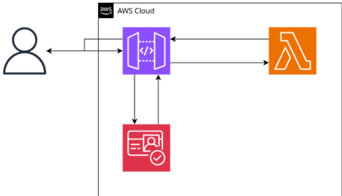
Figura 4: Schema del flusso di comunicazione tra Api Gateway, Lambda e Cognito [Elaborazione dell'autore]
