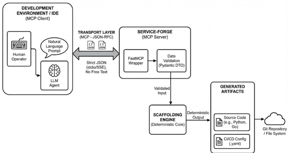
Figura 16: Architettura logica dell'integrazione MCP. Il diagramma illustra la separazione delle responsabilità tra l'IDE (Client MCP) delegato all'estrazione semantica tramite LLM, e Service-Forge (Server MCP) responsabile della validazione Pydantic e dell'esecuzione deterministica dello scaffolding [Elaborazione dell'autore].
