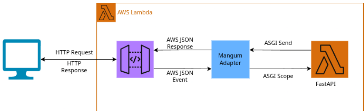
Figura 5: Schema del flusso di adattamento tramite Mangum. L'evento AWS viene tradotto in una richiesta compatibile con l'interfaccia ASGI [Elaborazione dell'autore]
