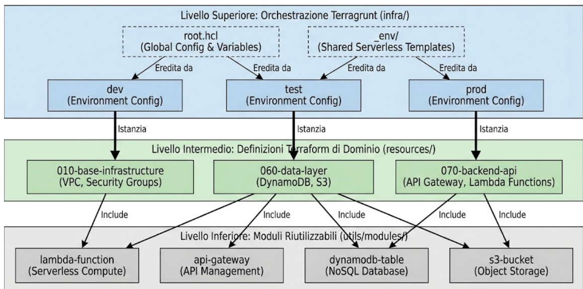
Figura 17: Architettura logica del repository di Infrastructure as Code. Il diagramma illustra la gerarchia di orchestrazione tra le configurazioni di ambiente gestite tramite Terragrunt (livello superiore), le definizioni dei domini funzionali (livello intermedio) e i moduli Terraform di base riutilizzabili (livello inferiore) [Elaborazione dell'autore].
