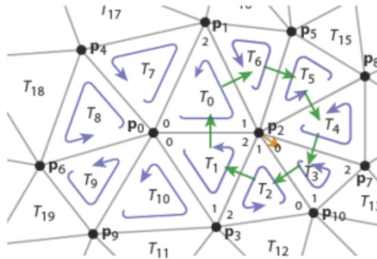
Figura 2.3: Rappresentazione della Triangle-Neighbor Structure : ogni triangolo referencia i tre triangoli adiacenti (uno per lato) e ogni vertice referencia uno dei triangoli incidenti.
