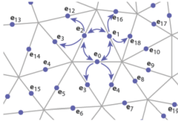
Figura 2.4: Rappresentazione della Winged-Edge Structure : ogni arco riferenzia i due vertici, le due facce adiacenti e gli archi successivo e precedente nella percorrenza di ciascuna faccia, assumendo la caratteristica forma a farfalla.
