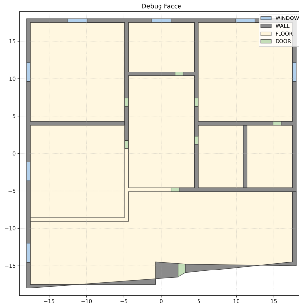
Figura 5.3: Facce estratte al primo tentativo: una faccia di muro non è classificata correttamente e sono presenti segmenti intrecciati in corrispondenza della porta d'ingresso.
