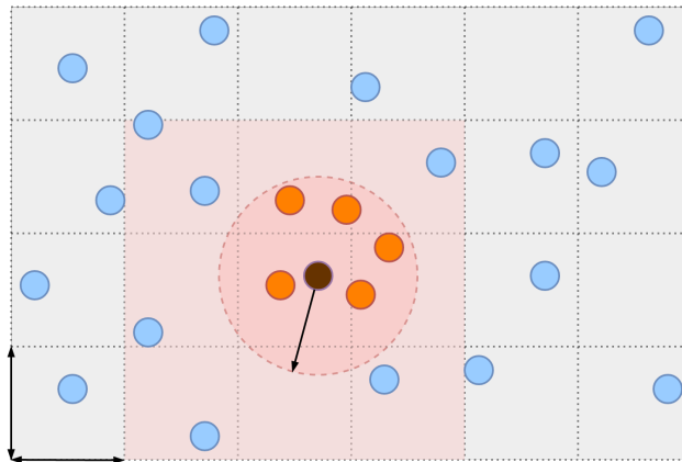
Figura 2.1: Rappresentazione di una griglia regolare per l'hash spaziale: i punti sono associati alle celle e la ricerca di prossimità esamina le celle adiacenti.
