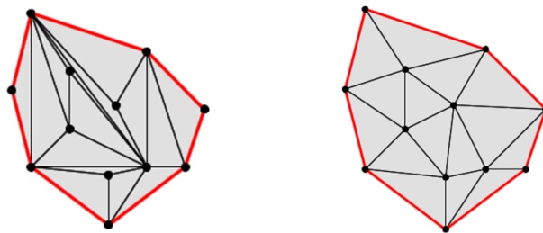
Figura 2.8: Confronto tra una connessione arbitraria dei punti e una triangolazione conforme al criterio di Delaunay. Nel secondo caso non ci sono triangoli degeneri.
