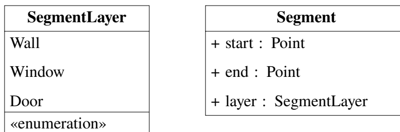
Figura 3.4: Diagramma UML delle entità Segment e SegmentLayer, che rappresentano rispettivamente un segmento geometrico e la sua semantica (muro, porta o finestra).
