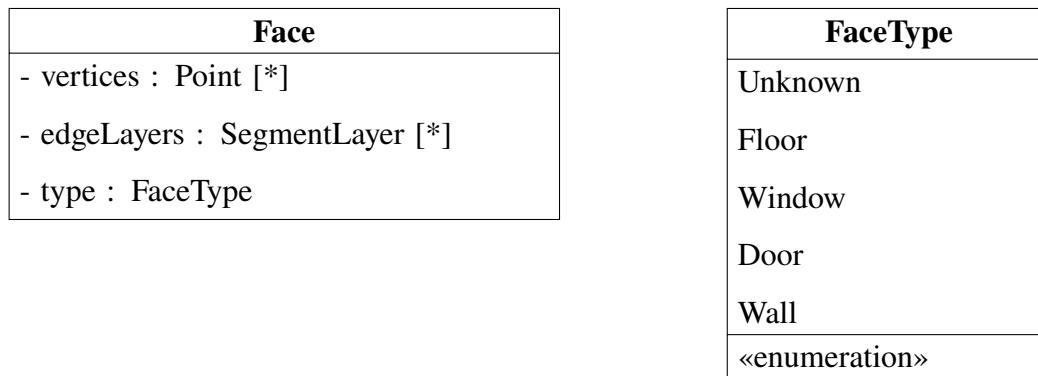
Figura 3.13: Diagramma UML della classe Face, che rappresenta una faccia del grafo con i relativi vertici, la semantica degli archi e il tipo di faccia.
