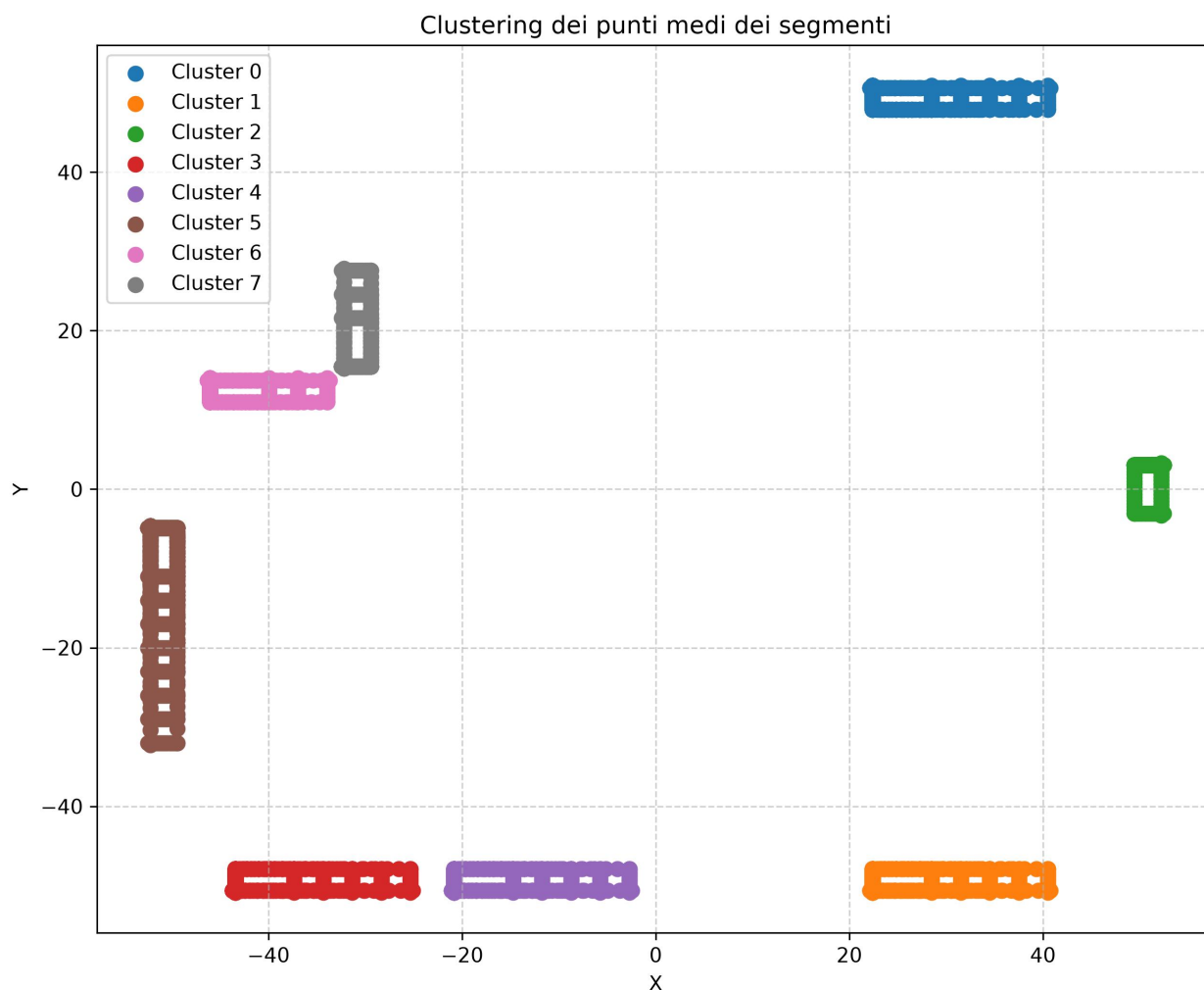
Figura 3.11: Cluster dei punti delle finestre individuati da DBSCAN con \text{num\_samples} = 15 e \epsilon = 2 .
