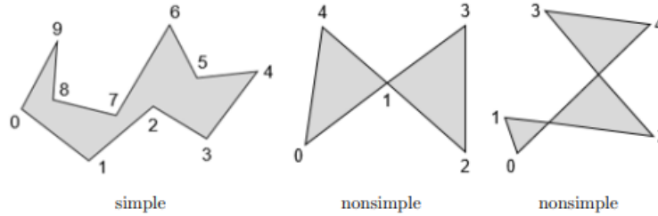
Figura 2.6: Rappresentazione di un poligono semplice: i vertici sono collegati in sequenza da spigoli che non si intersecano se non nei vertici stessi.
