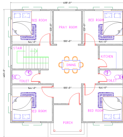
Figura 5.10: Modello CAD del terzo caso di studio.
