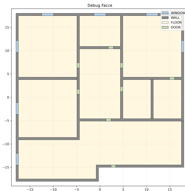
Figura 5.6: Facce estratte dopo le correzioni: la classificazione è corretta.
