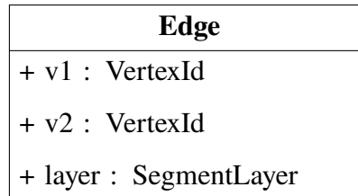
Figura 3.8: Diagramma UML della struttura Edge, che rappresenta un lato del grafo con la relativa semantica.
