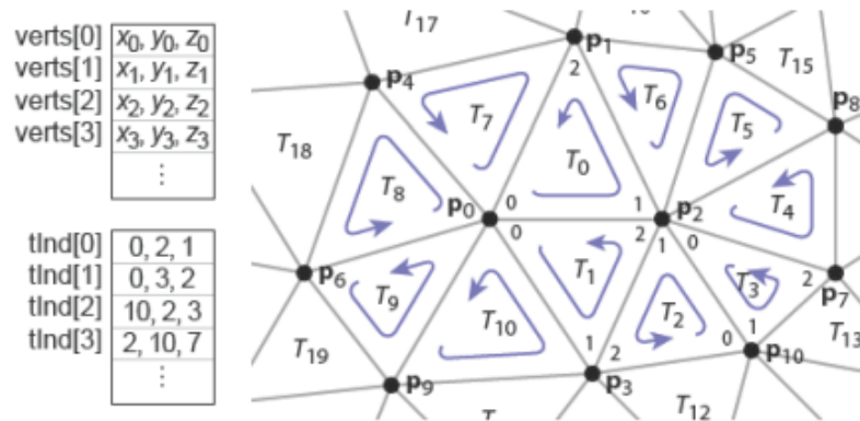
Figura 2.2: Rappresentazione di una indexed triangle mesh : i vertici sono memorizzati una sola volta e ogni triangolo vi fa riferimento tramite indici.
