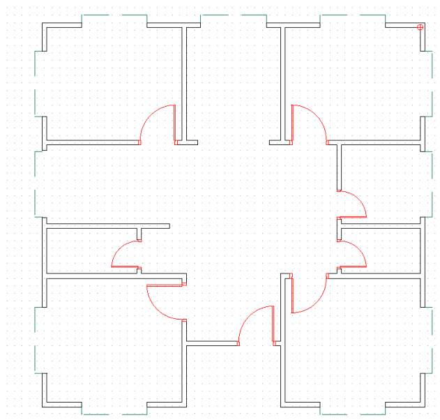
Figura 5.11: Modello CAD dopo la creazione manuale dei varchi per le finestre.
