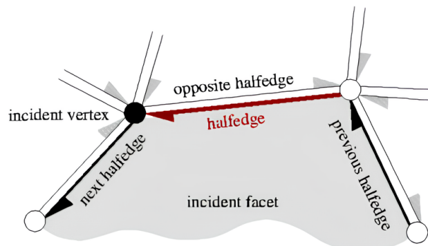
Figura 2.5: Rappresentazione della Half-Edge Structure : ogni arco è suddiviso in due half-edge opposti, ciascuno con riferimenti alla faccia, al vertice di destinazione, al gemello e all'half-edge successivo.
