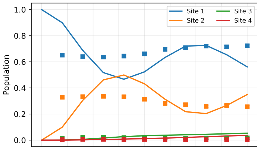
mit Reset (Mid-Circuit) (60 Kreise, t=1..10 )
