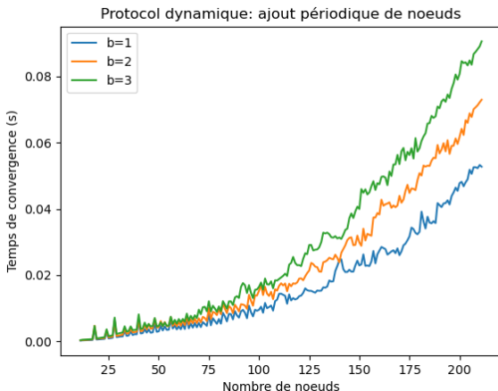
Figure – Ajout successifs de 180 noeuds à partir de |R| = 20
