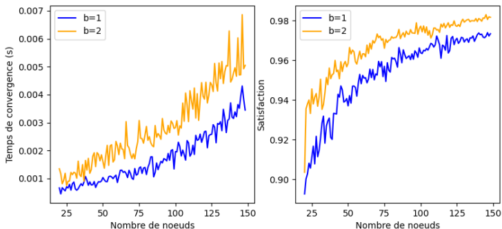
Figure – Ajout et retrait successifs à |R| fixé
