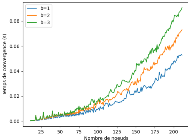
Figure – Ajout successifs de 200 noeuds à partir de |R| = 10
