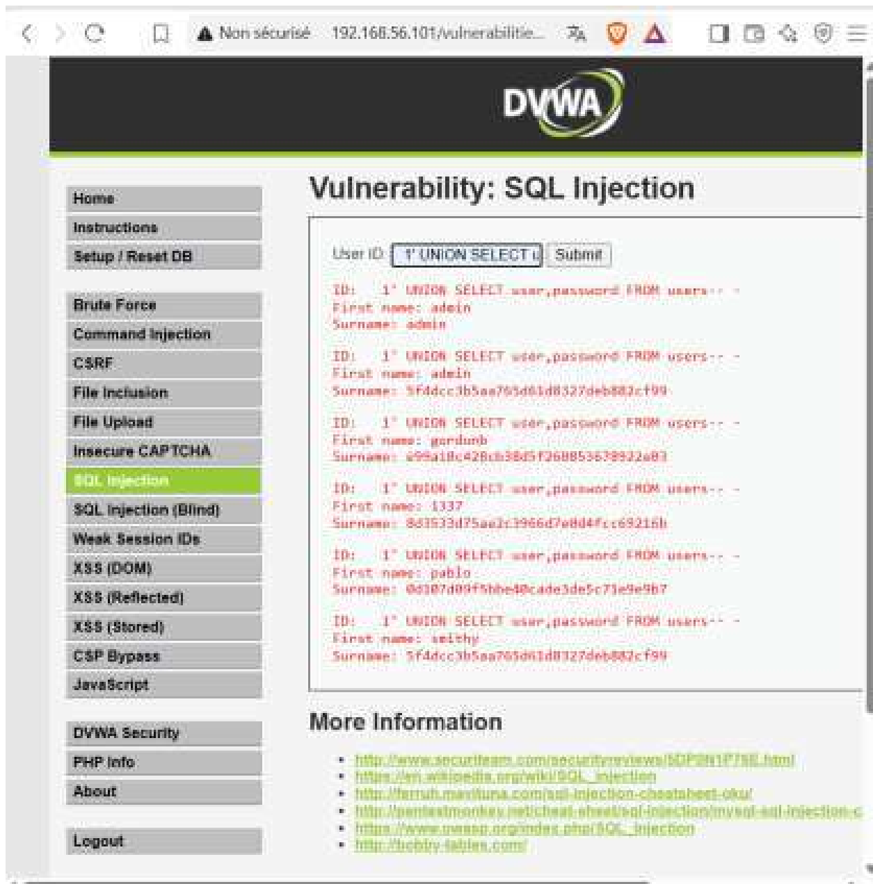
Figure 30: Résultat de l'injection UNION dans DVWA : comptes et hachés MD5 affichés.
