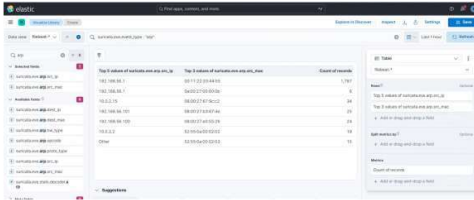
Figure 26: Table Kibana : 192.168.56.1 associée à deux adresses MAC.
