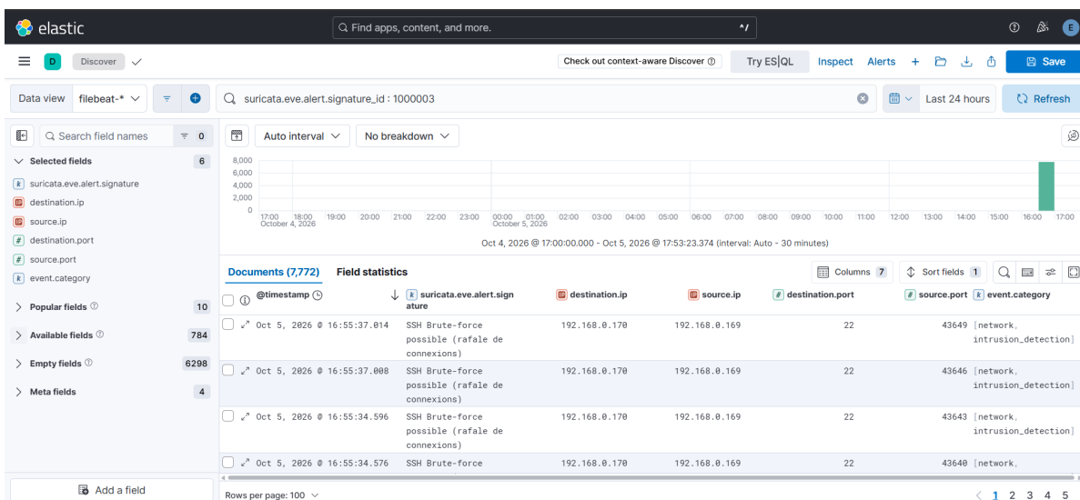
Figure 20: Visualisation du brute-force SSH dans Kibana
