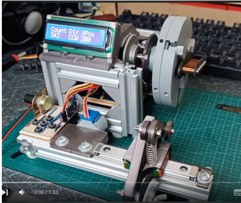
Abbildung 4: Screenshot vom Open Source Pickup Winder
