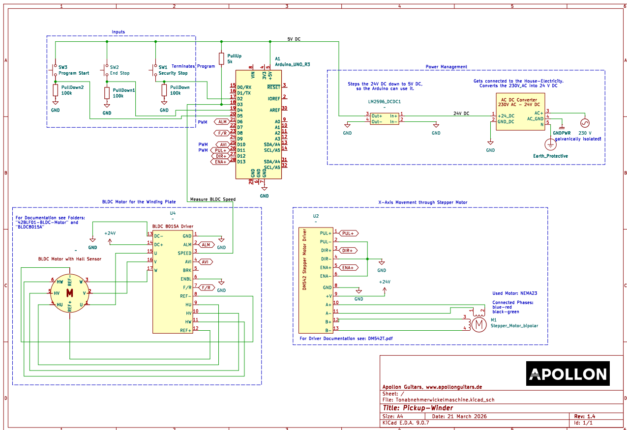
Abbildung 5: Schaltplan aus Circuit-Design/Tonabnehmerwickelmaschine_Schaltplan.pdf
