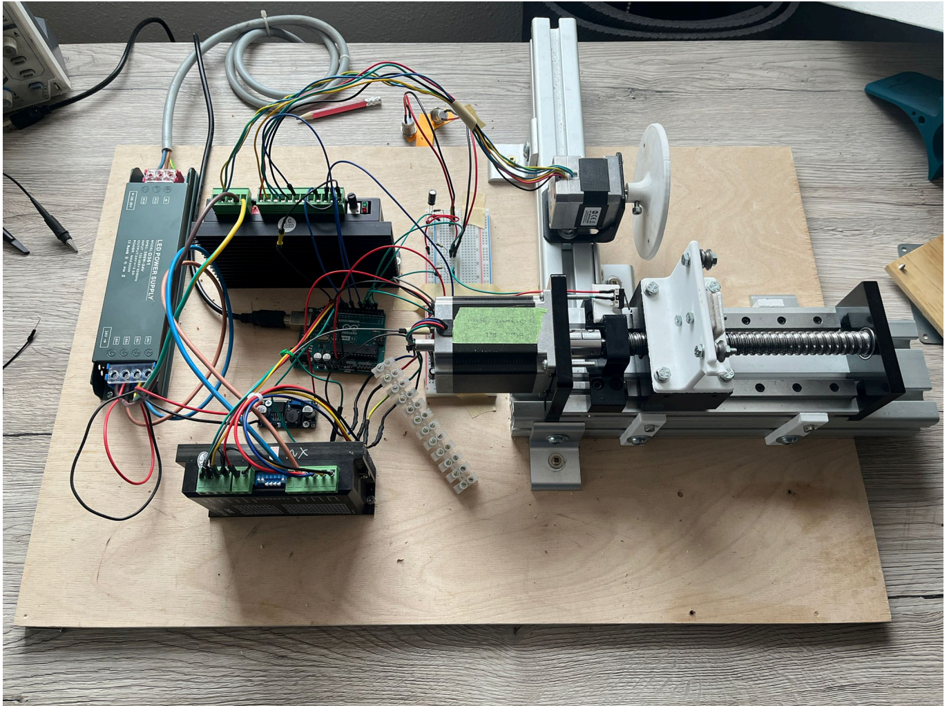
Abbildung 1: Die Tonabnehmerwickelmaschine
