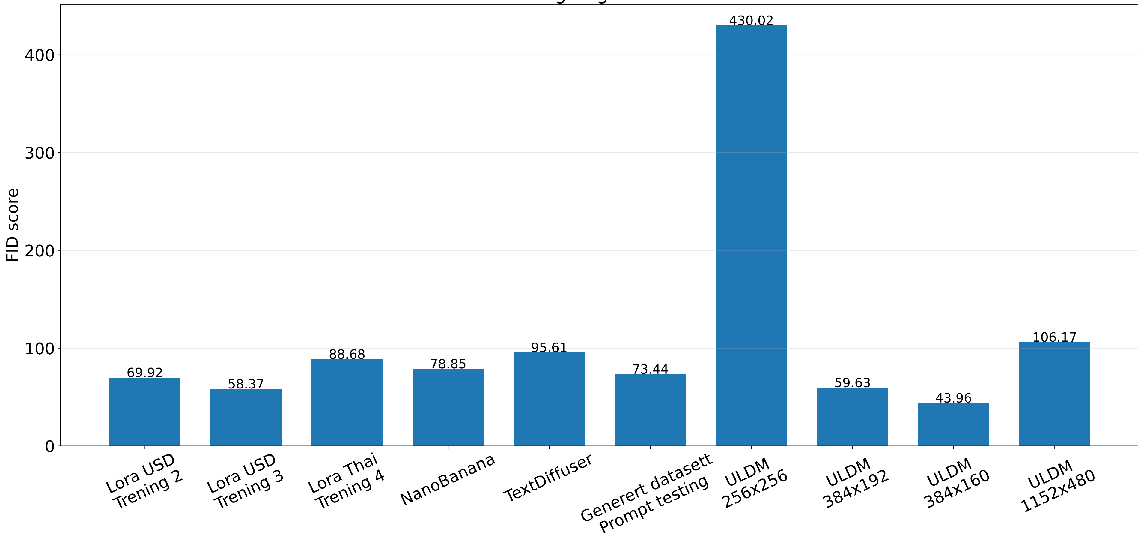
FID sammenligning av ulike metoder
