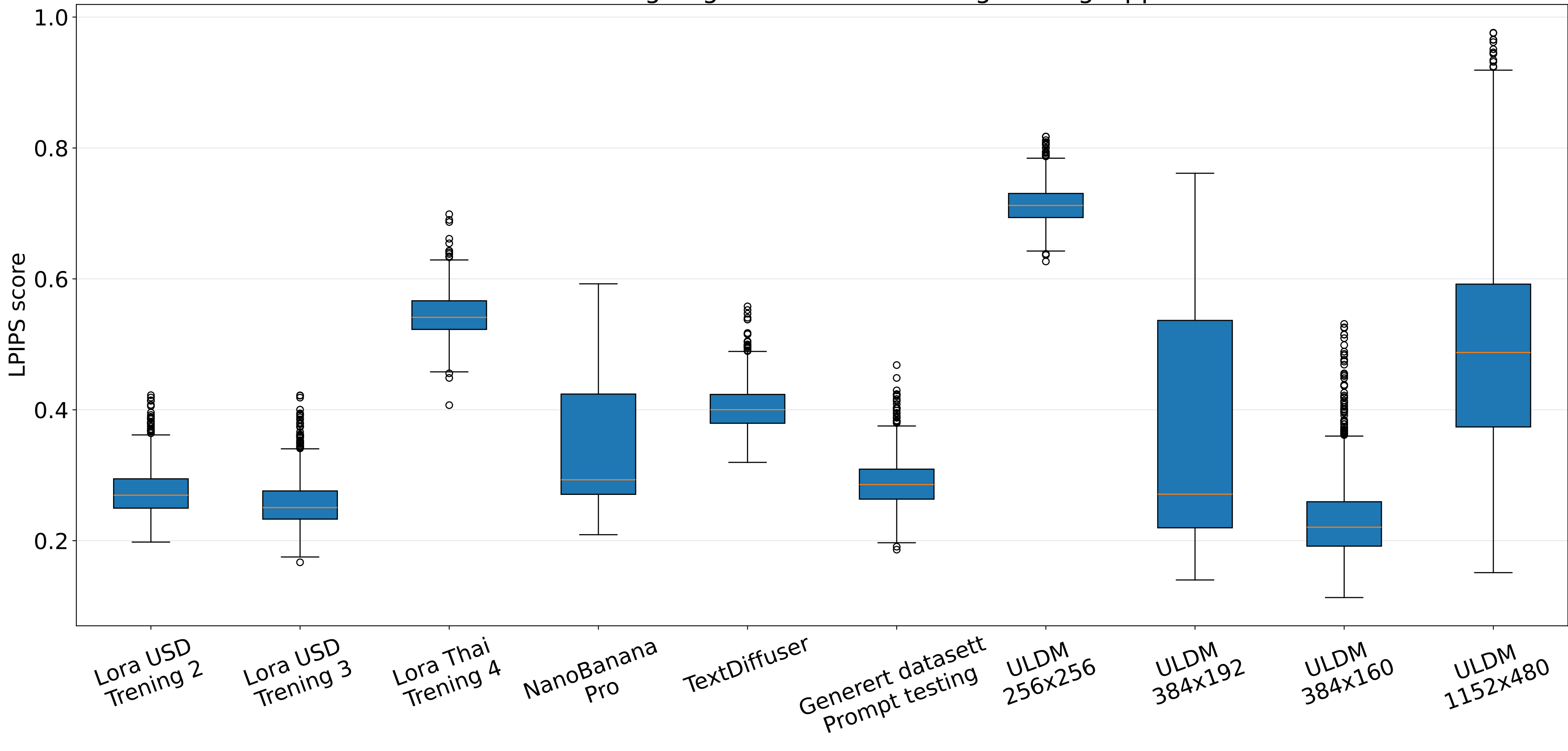
LPIPS sammenligning av ulike metoder og treningsoppsett
