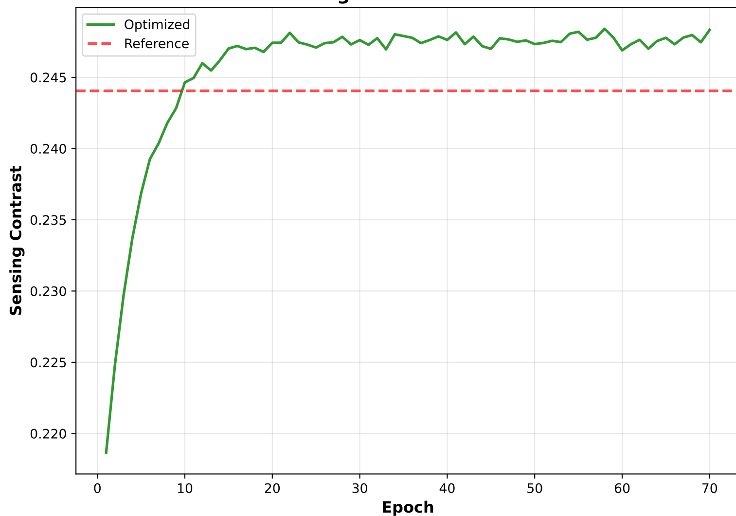
Parameter Evolution
