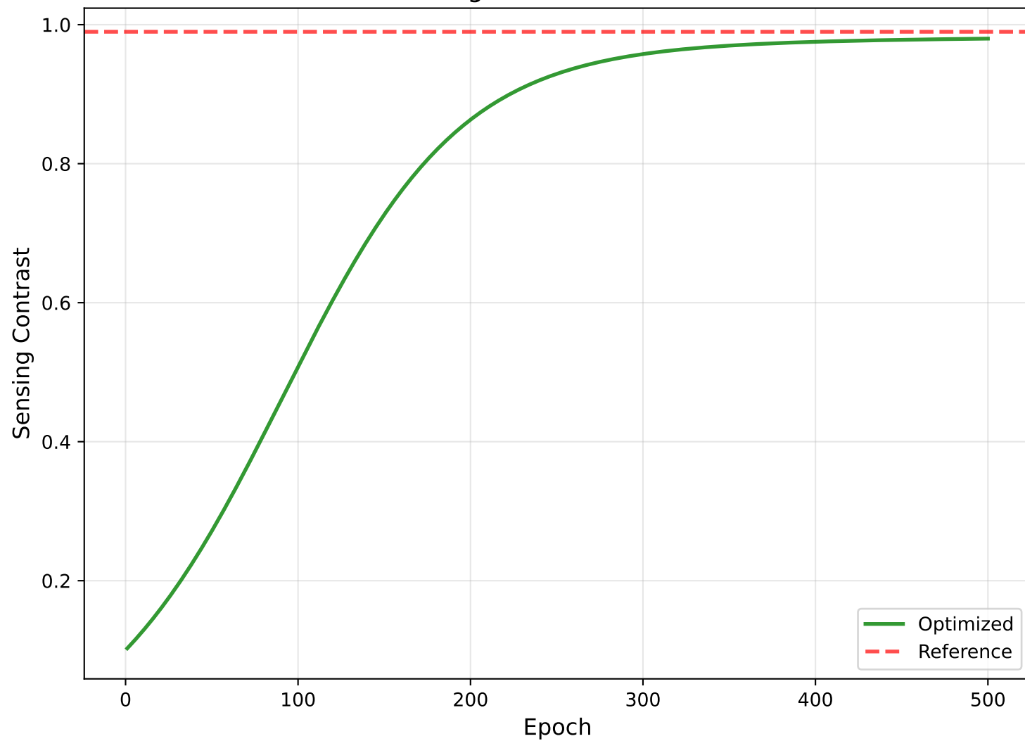
Parameter Evolution
