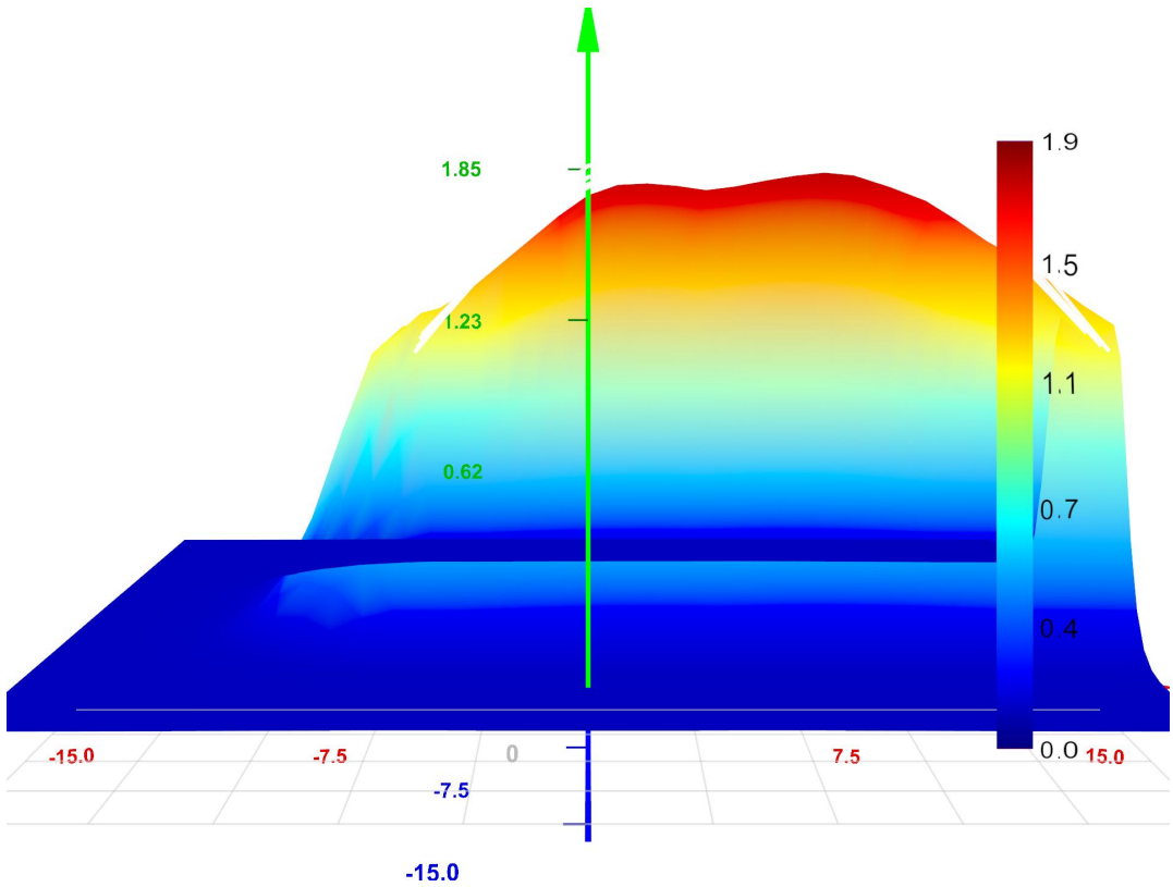
图 3：主视图 (X-B 切面轴向磁场曲线)
