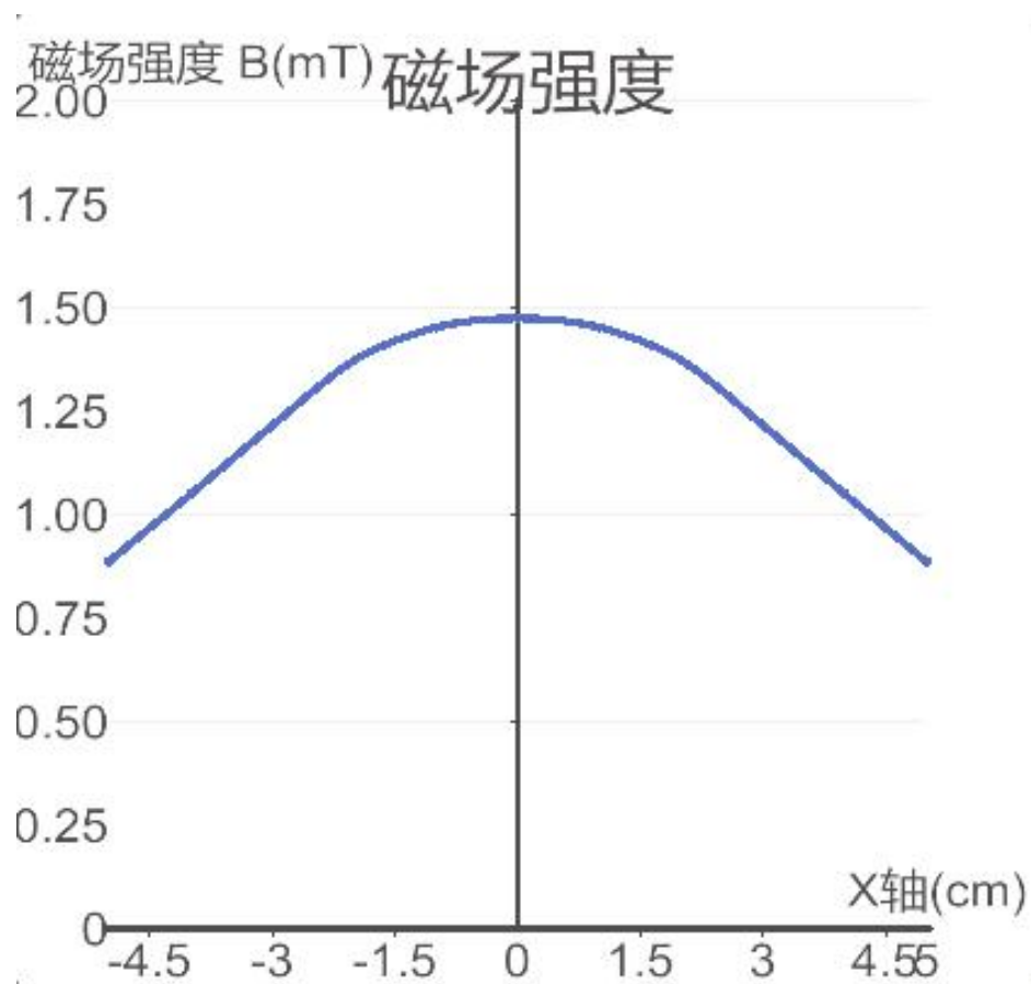
二、磁场空间分布图 ( f = 50.0 \text{ Hz} , I = 1.0 \text{ mA} )
