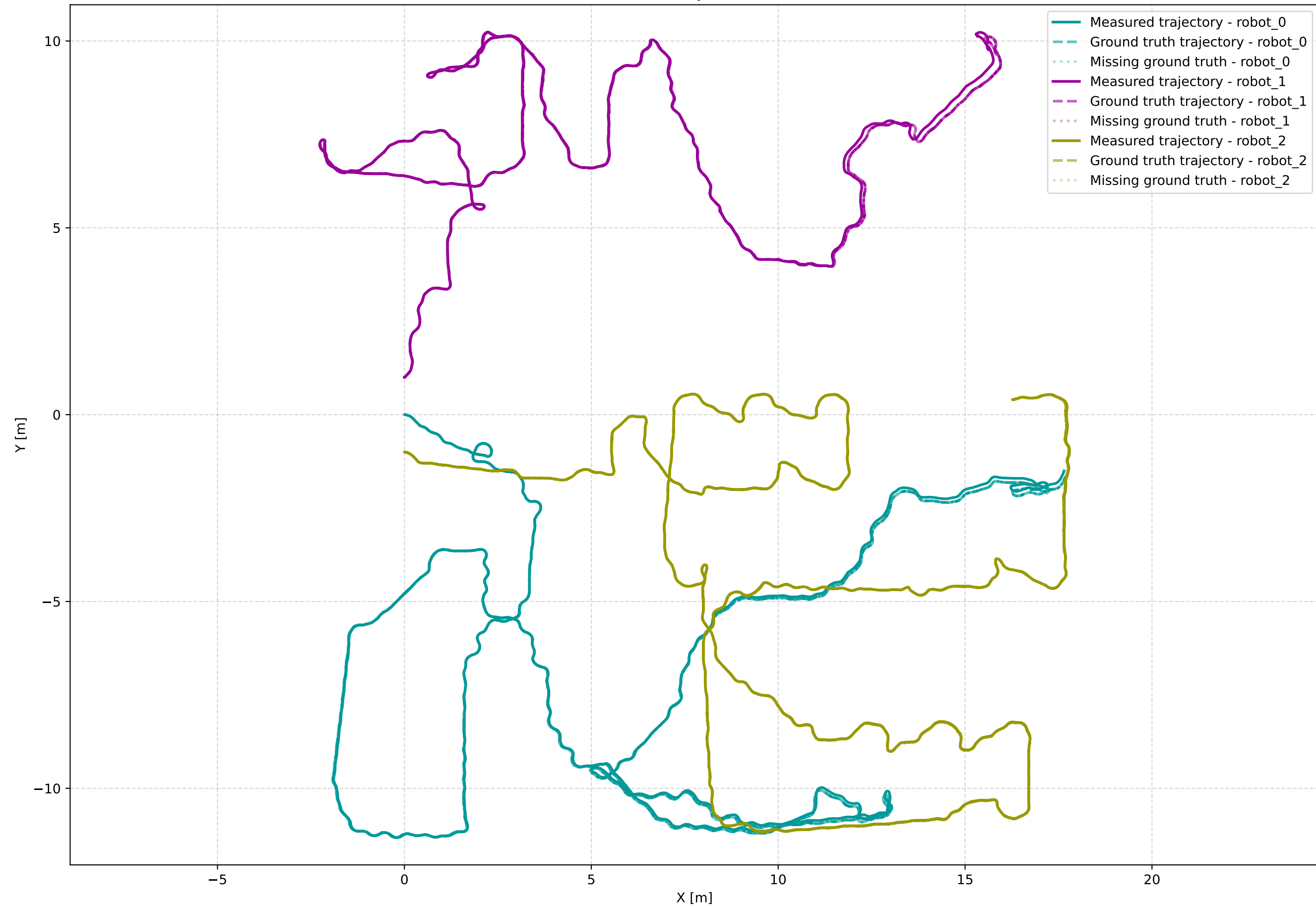
Robot trajectories
