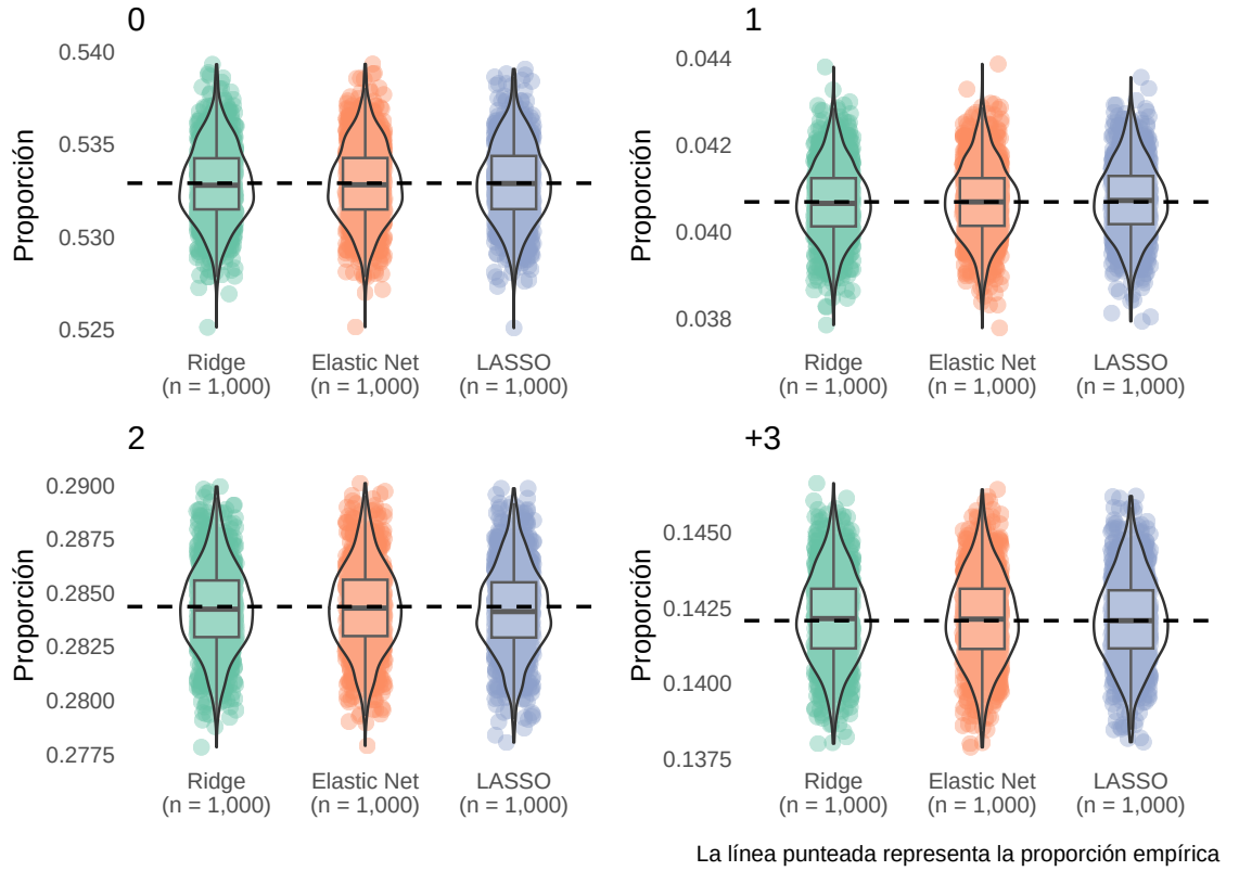
Figura 18: Simulación de distribución empírica
