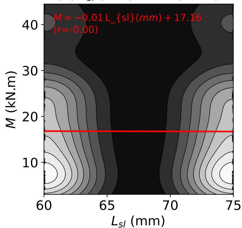
(d) L_{sl} (mm) vs. M (kN.m)
