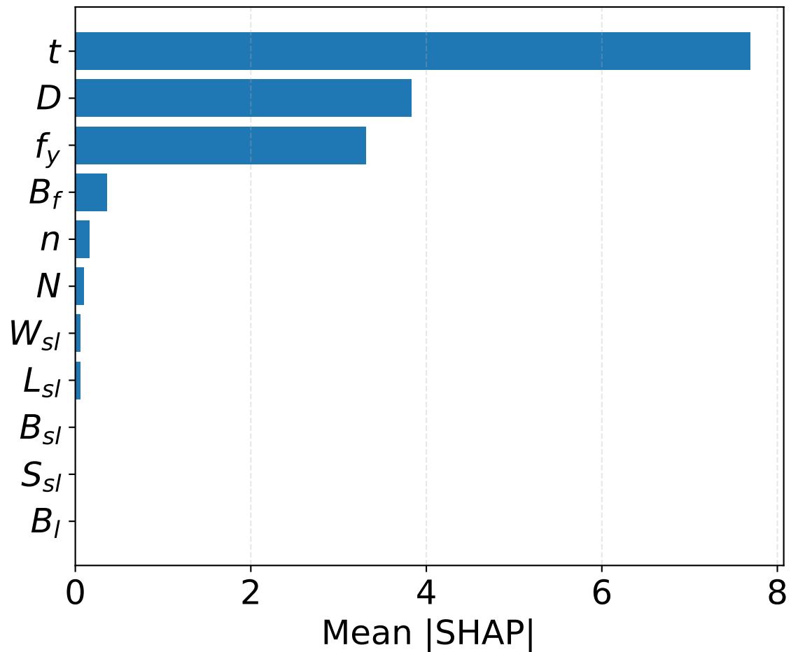
(b) Mean absolute SHAP values
